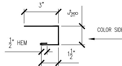
C-METAL TRIM (WS-1601)
