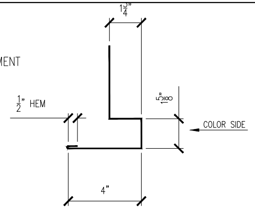
SILL DRIP TRIM (WS-1604)
