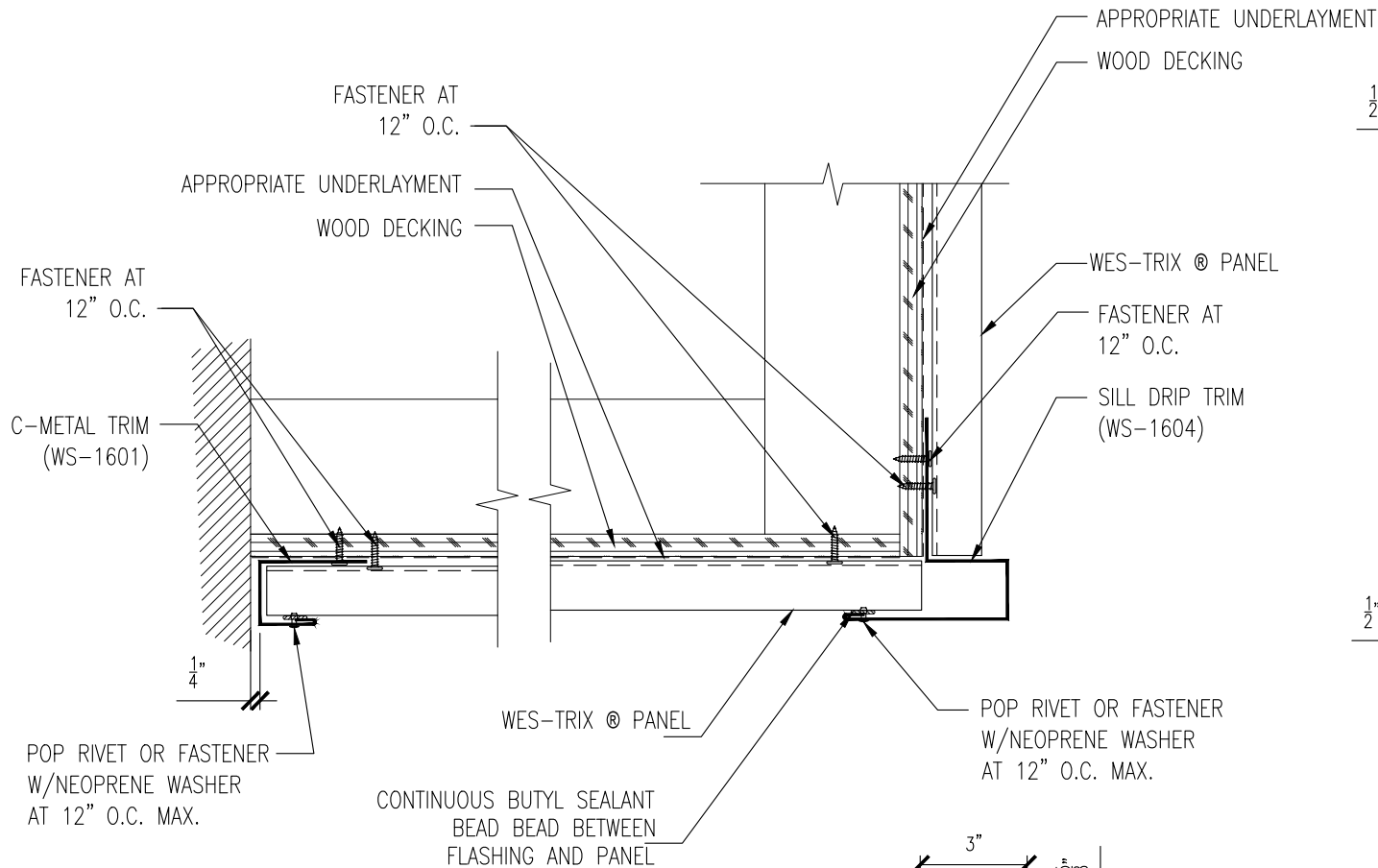
SILL DRIP TRIM (WS-1604)
