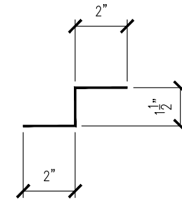
Z-METAL TRIM (WS-1606)
